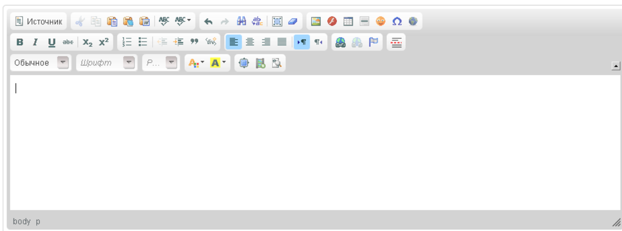
Рисунок 1.1 – Интерфейс редактора
