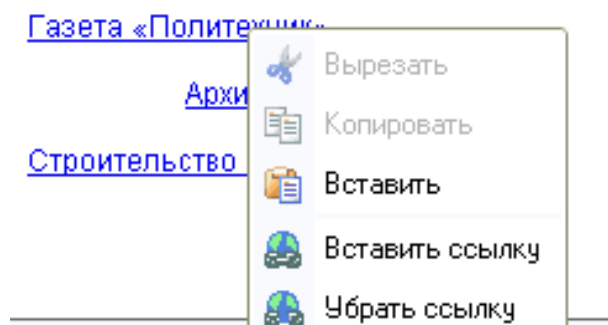
Рисунок 4.1 – Контекстное меню
